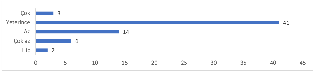
Şekil 7. Endüstri mühendisliği hakkındaki bilgi seviyesinin grafiksel gösterimi
