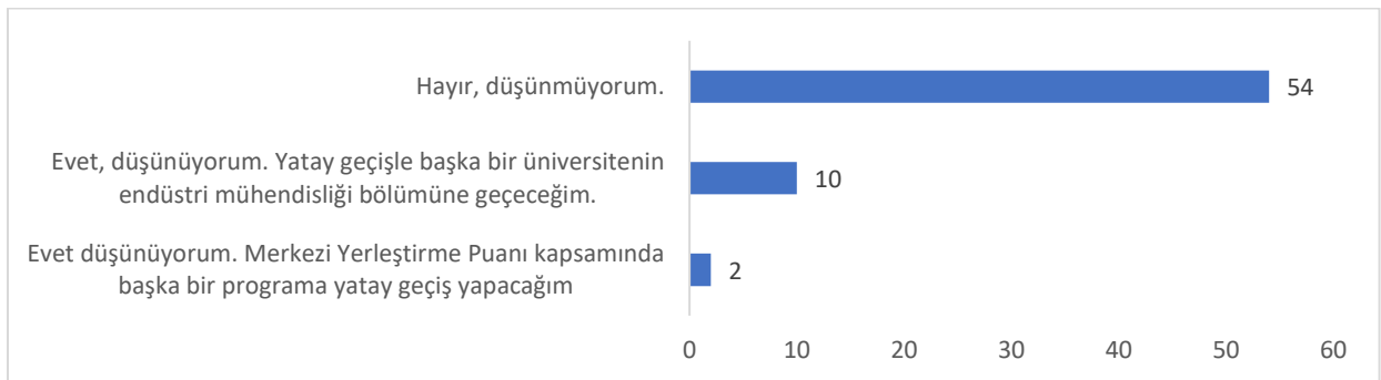
Şekil 14. Öğrencilerin üniversite değişikliği hakkındaki fikirlerinin grafiksel gösterimi
