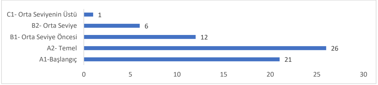
Şekil 15. Yabancı dil seviyesi grafiksel gösterimi
