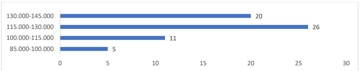
Şekil 3. Öğrenci sıralamalarının grafiksel gösterimi
