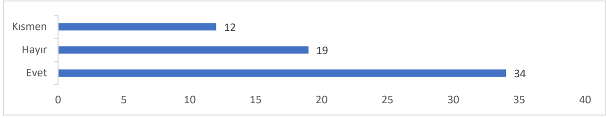
Şekil 11. MÜDEK grafiksel gösterim
