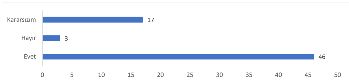
Şekil 10. EMMT katılım isteği grafiksel gösterim
