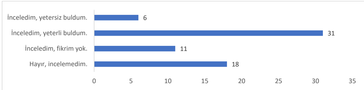
Şekil 8. Web sayfası incelemesinin grafiksel gösterimi
