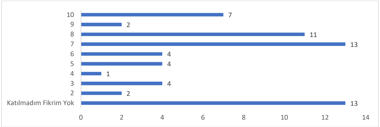
Şekil 16. Oryantasyon programı değerlendirmesi
