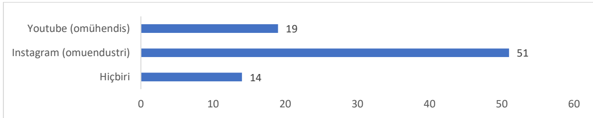
Şekil 9. Sosyal medya araçları grafiksel gösterim
