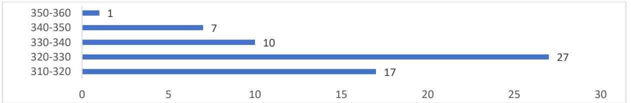
Şekil 2. Öğrenci puanlarının grafiksel gösterimi
