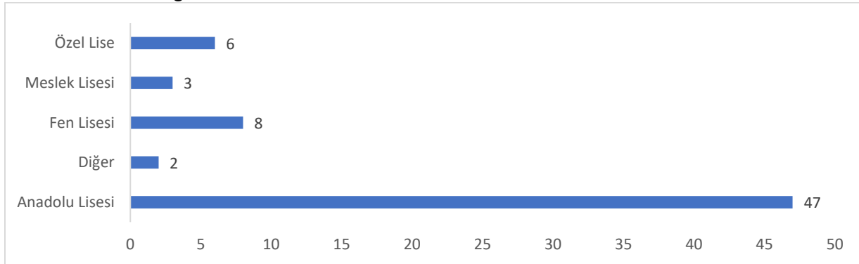
Şekil 6. Mezun olunan lise türünün grafiksel gösterimi
