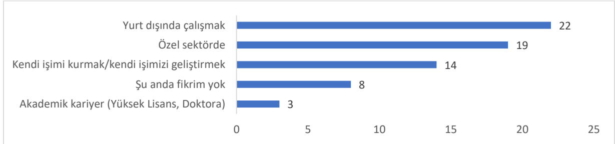
Şekil 13. Öğrencilerin kariyer hedeflerinin grafiksel gösterimi
