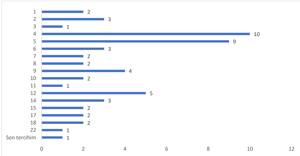
Şekil 5. Endüstri Mühendisliği ve OMÜ Endüstri Mühendisliğini seçen öğrencilerin karşılaştırılması
